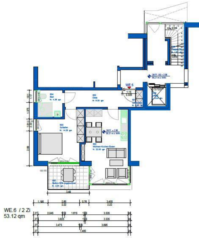
1. Obergeschoss WE 06
